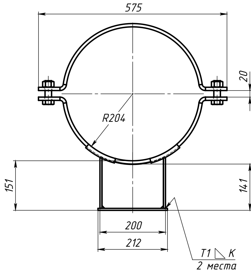
Поз.4 (Полухомут)
