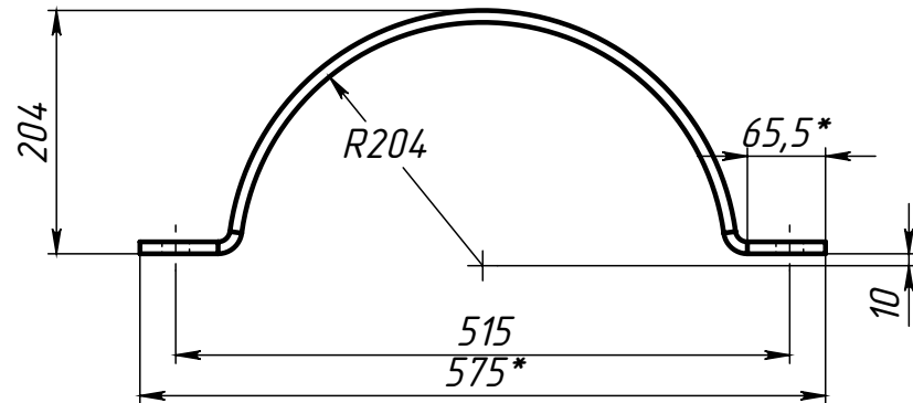
Поз.4 (Полухомут)
